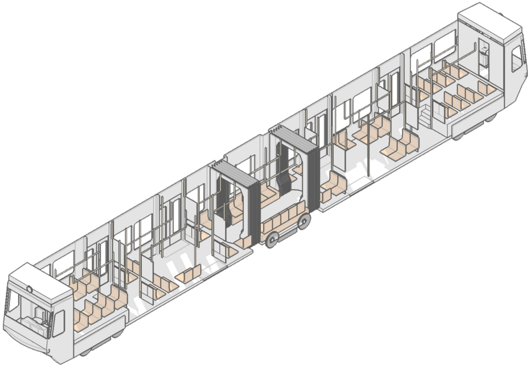
TRIMET MAX Type II
